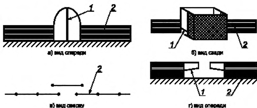
1 — штанга против велосипедов; 2 — ограждение универсального спортивного оборудования
