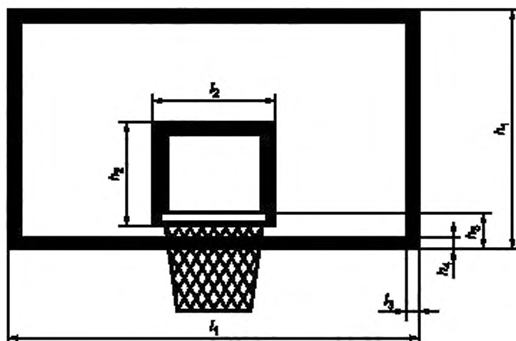
Рисунок 8 — Рекомендуемые размеры баскетбольного щита и размеры маркировки
