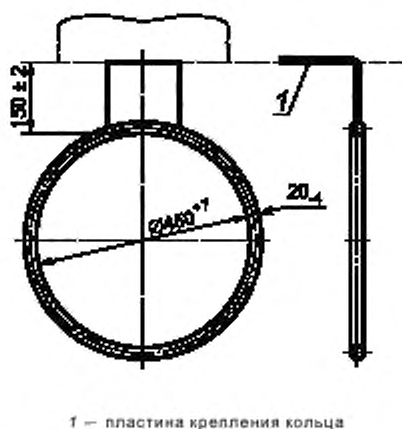
Рисунок 9 — Размеры баскетбольного кольца
