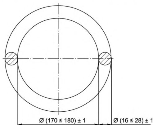
Рисунок 2 — Размеры гимнастического кольца
