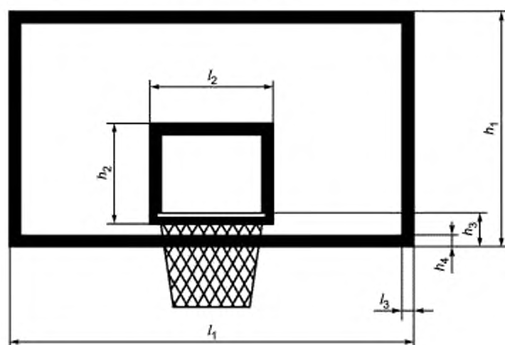
Рисунок 3 — Размеры и разметка баскетбольного щита
