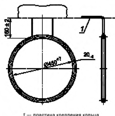
Рисунок 5 — Размеры баскетбольного кольца
