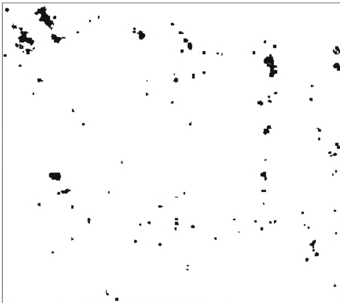
Рисунок Ж.3 — Коррозия металла балл К3 (или Rі 3)
