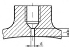
Рисунок 8 – Пример разъема для измерения давления
