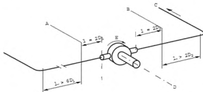
А – точка измерения избыточного давления на входе; В – точка измерения избыточного давления на выходе; С – к прибору измерения Q и нагнетательному клапану; D – вал двигателя – горизонтальный; E – направление потока; D_1 – внутренний диаметр трубы и входа насоса; D_2 – внутренний диаметр трубы и выхода насоса
