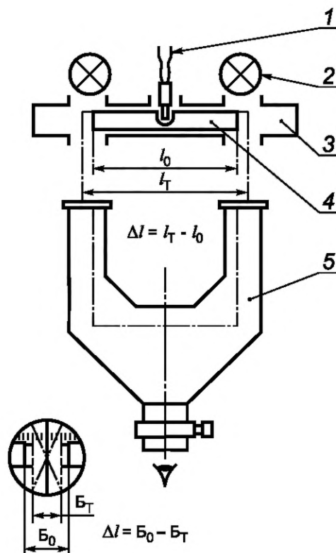
1 — термопара; 2 — осветитель; 3 — нагреватель; 4 — испытываемый образец; 5 — микроскоп-компаратор
