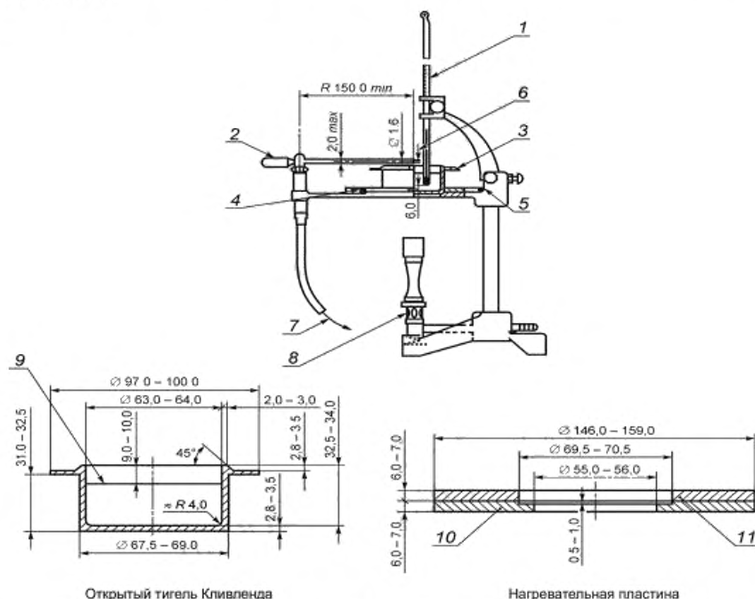
1 — термометр; 2 — зажигательное устройство; 3 — тигель; 4 — металлический шарик диаметром от 3,2 до 4,8 мм; 5 — нагревательная пластина; 6 — отверстие диаметром 0,8 мм; 7 — к источнику газа; 8 — нагревательный прибор пламенного типа или резистивный электронагреватель; 9 — отметка заполнения; 10 — металлическая пластина; 11 — теплостойкая пластина
