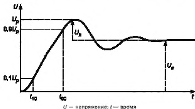
Рисунок 1 — Параметры импульса напряжения
