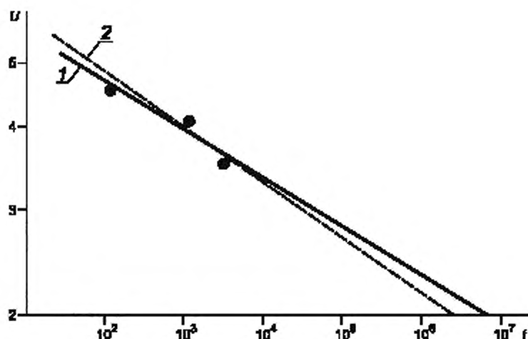
1 — срок службы межвитковой изоляции; 2 — срок службы корпусной изоляции; f — время до пробоя, U = U_{испыт}/U_{итп} — для витковой изоляции; U = U_{испыт}/U_{ном} — для корпусной изоляции
