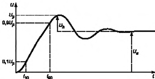
Рисунок 1 — Параметры импульса напряжения
