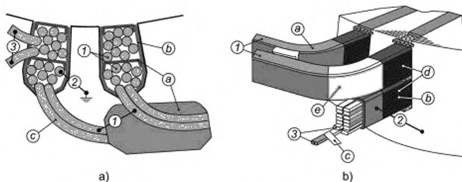
a — фазная изоляция (межслойная); b — изоляция на землю; c — витковая изоляция; d — система защиты от короны в лазу; e — система выравнивания напряженности электрического поля; 1 — межфазная изоляция; 2 — изоляция «фаза—земля»; 3 — межвитковая изоляция
