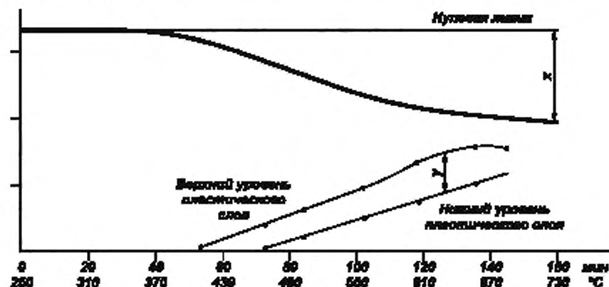
Рисунок 6 — Пологопадающая кривая
