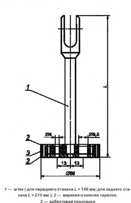
Рисунок 3 — Штемпель
