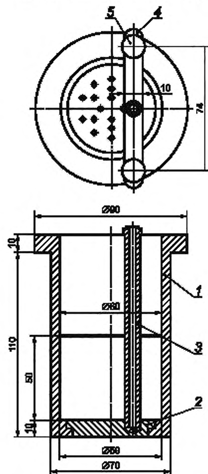
1 — корпус; 2 — доншко; 3 — трубка для термопары; 4 — прижимная планка; 5 — прижимной винт
