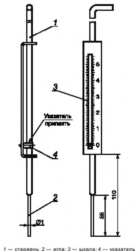
Рисунок 4 — Игла-пластометр
