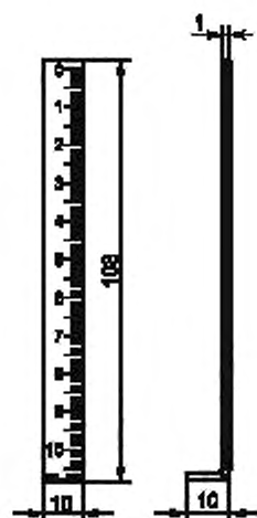
Рисунок В.1 — Линейка
