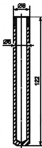
Рисунок 2б — Трубка для термопары
