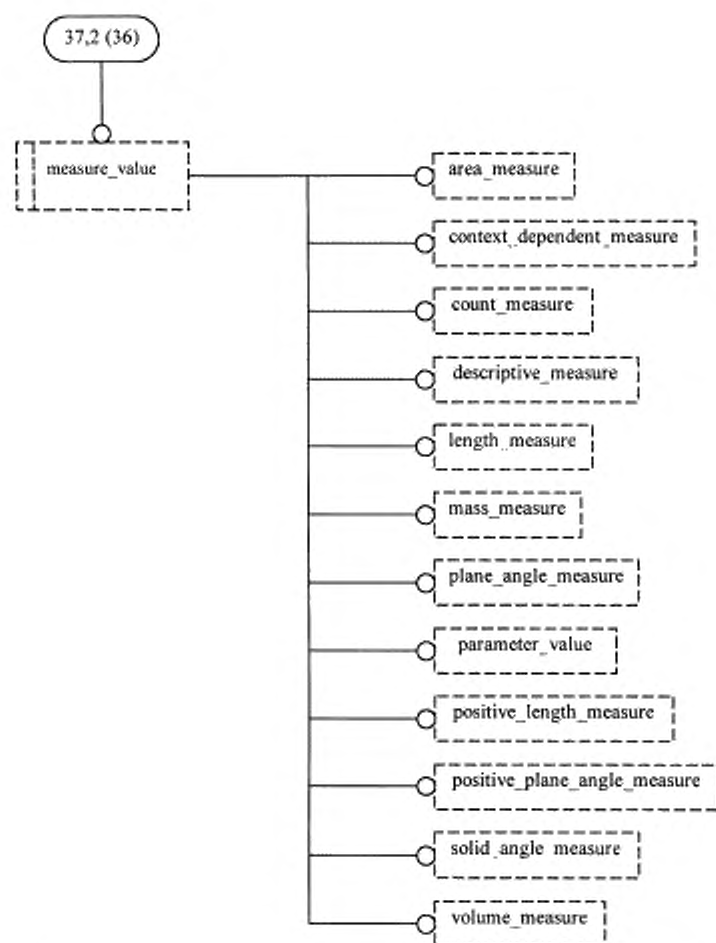
Рисунок Н.37 — measures — ПИМ EXPRESS-G диаграмма 37 из 39
