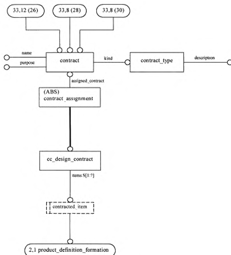
Рисунок Н.33 — contract — ПИМ EXPRESS-G диаграмма 33 из 39
