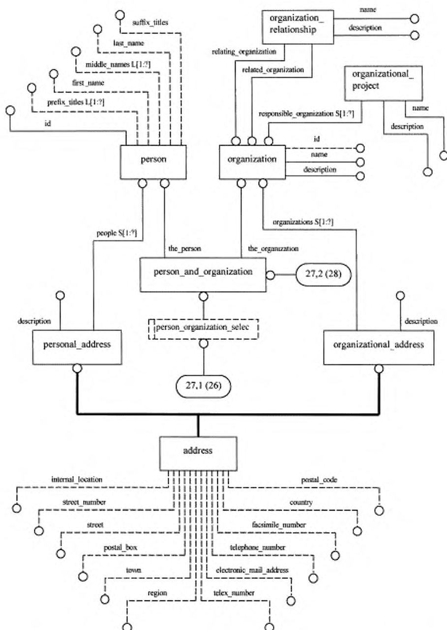
Рисунок Н.27 — person_and_organization — ПИМ EXPRESS-G диаграмма 27 из 39
