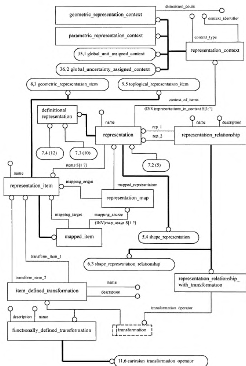
Рисунок Н.7 — representation — ПИМ EXPRESS-G диаграмма 7 из 39
