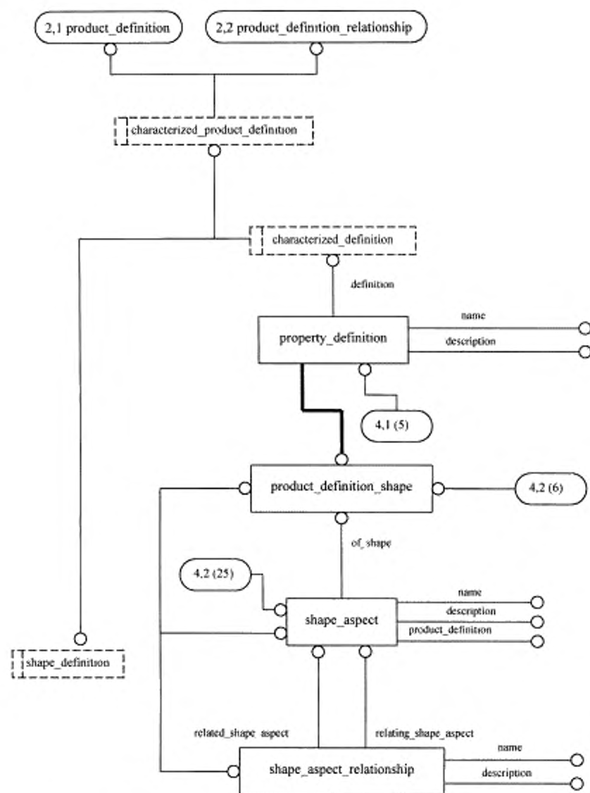
Рисунок Н.4 — property_definition — ПИМ EXPRESS-G диаграмма 4 из 39
