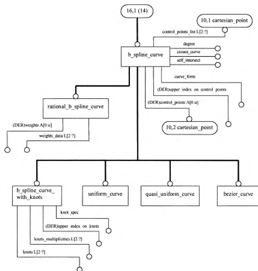
Рисунок Н.16 — b_spline_curve — ПИМ EXPRESS-G диаграмма 16 из 39
