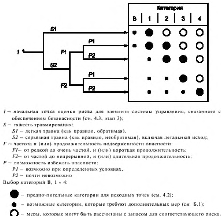
Рисунок Б.1 — Выбор категорий для элементов систем управления, связанных с обеспечением безопасности
