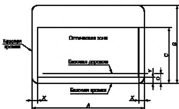
Рисунок 1 — Размеры и расположение оптической зоны
