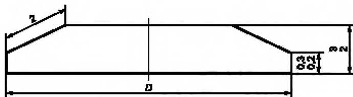
Рисунок Д.2 — Калибровочный диск
