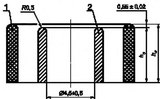
1 — сменная подложка для очковых линз высотой h_c ; 2 — подложка для контактных линз высотой h_c
