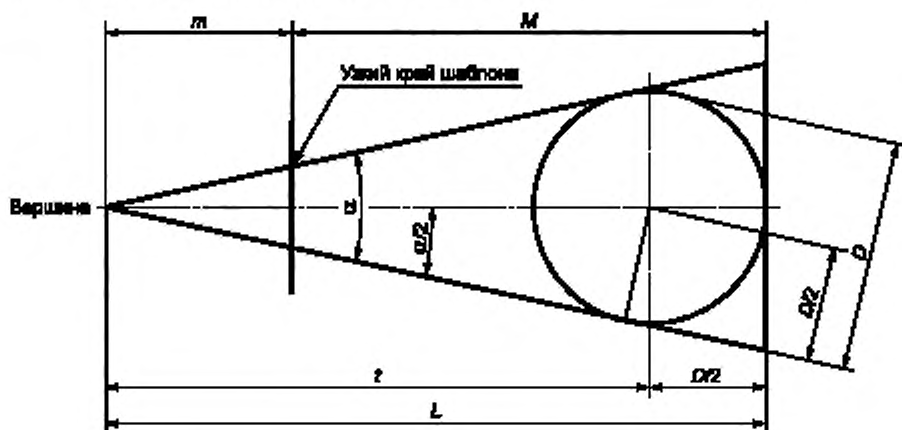
Рисунок Д.3 — Геометрические соотношения для V-образного шаблона
