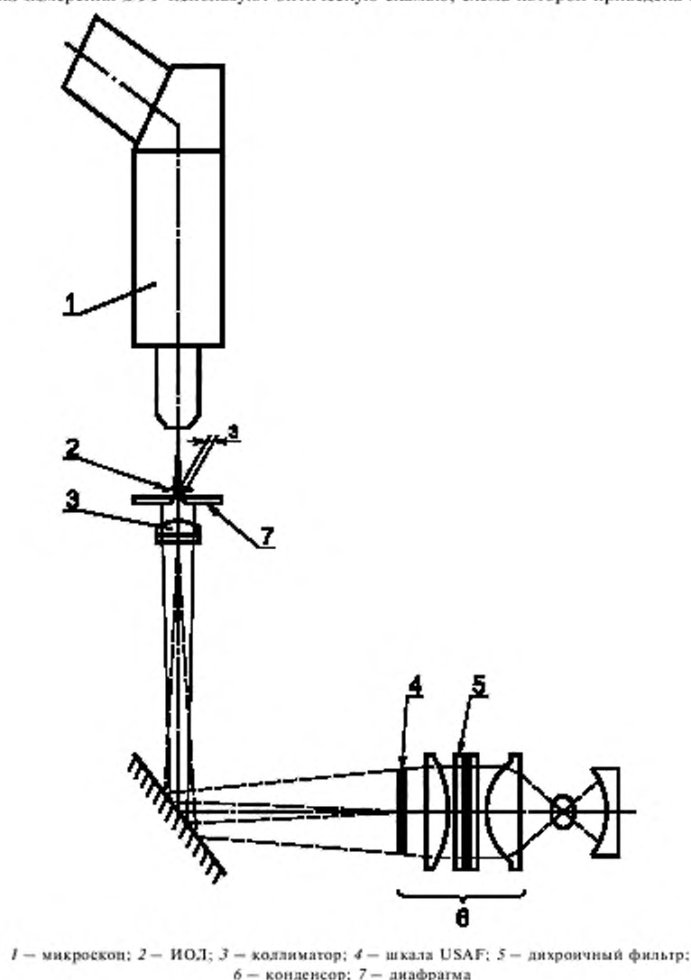
Рисунок А.1 — Оптическая скамья с ИОЛ
