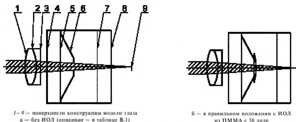
Рисунок В.1 — Модель глаза
