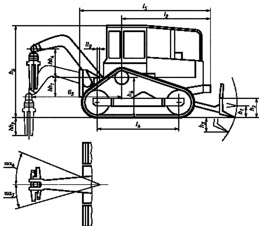
Рисунок 6 — Трелевочная машина с ланковым захватом на базе промышленного шасси. Основные размеры в продольной вертикальной плоскости
