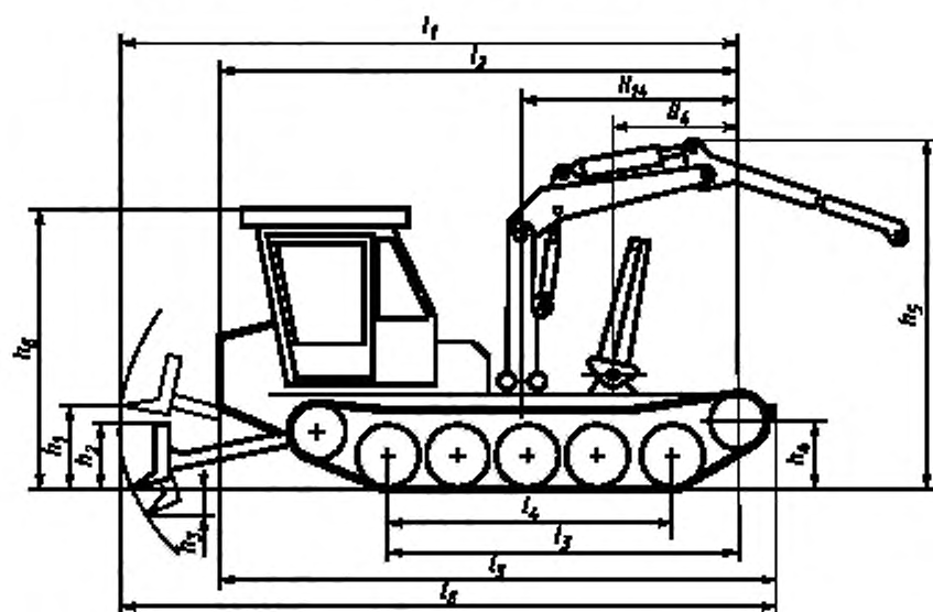
Рисунок 8 — Трельовочная машина с манипулятором и ковшом (часть вилки верхнего раствора). Размеры в продольной вертикальной плоскости
