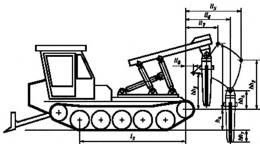
Рисунок 3 — Трепавочная машина с пачковым захватом (челюстями нижнего раствора) на базе конструкции параллелограммного механизма. Размеры захвата в вертикальной плоскости
