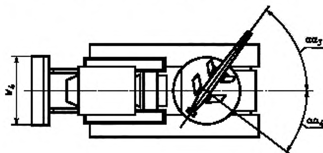
Рисунок 4 — Трепавочная машина с челюстями нижнего раствора. Вид сверху по рисунку 3 (захват не показан)
