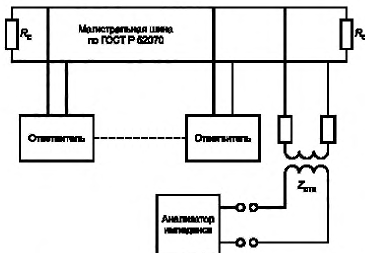
Рисунок 3 — Измерение импеданса ответвителя с трансформаторной связью
