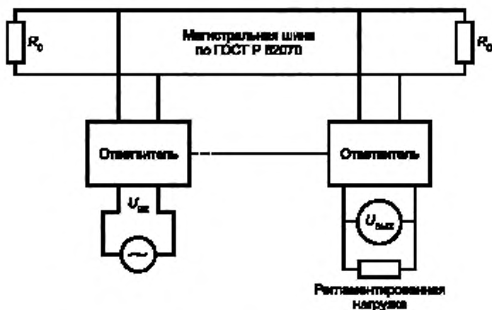
Рисунок 5 — Измерение затухания в магистральной шине/ответвителе
