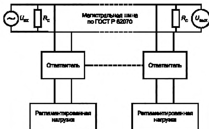
Рисунок 4 — Измерение затухания в магистральной шине
