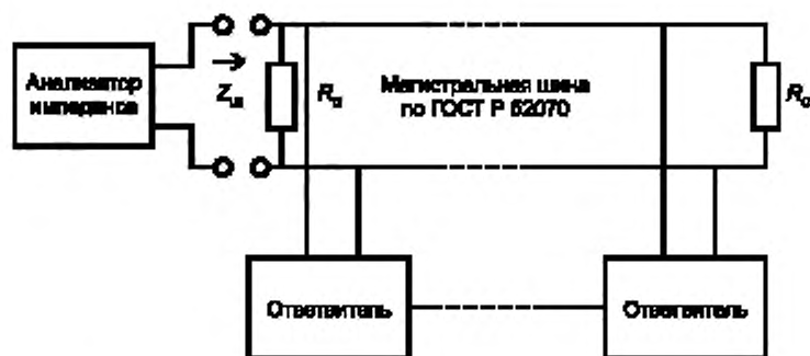
Рисунок 2 — Измерение импеданса магистральной шины
