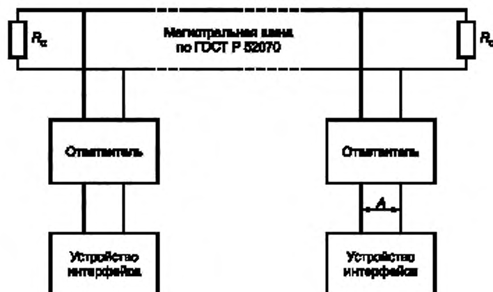
Рисунок 1 — Измерение активного сопротивления ответвителя с трансформаторной связью
