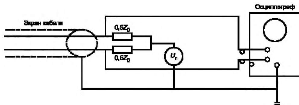
Рисунок 7 — Схема тестирования передачи при воздействии синфазных помех
