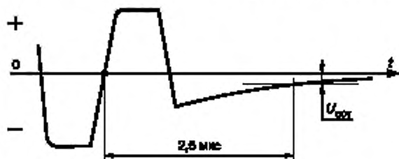
Рисунок 9 — Симметрия сигнала
