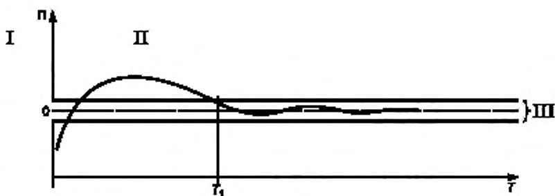
I — питание выключено; II — питание включено; III — пределы допускаемых отклонений показания прибора в чистом воздухе; P — показание; T — время; 0 — ноль прибора; T_1 — время прогрева (см. 2.6.7)
