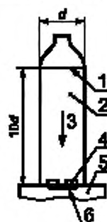
1 — диффузионный барьер; 2 — трубчатый аппликатор; 3 — поток чистого воздуха или ПГС; 4 — емкость; 5 — прибор или датчик; 6 — входное отверстие прибора (датчика)
