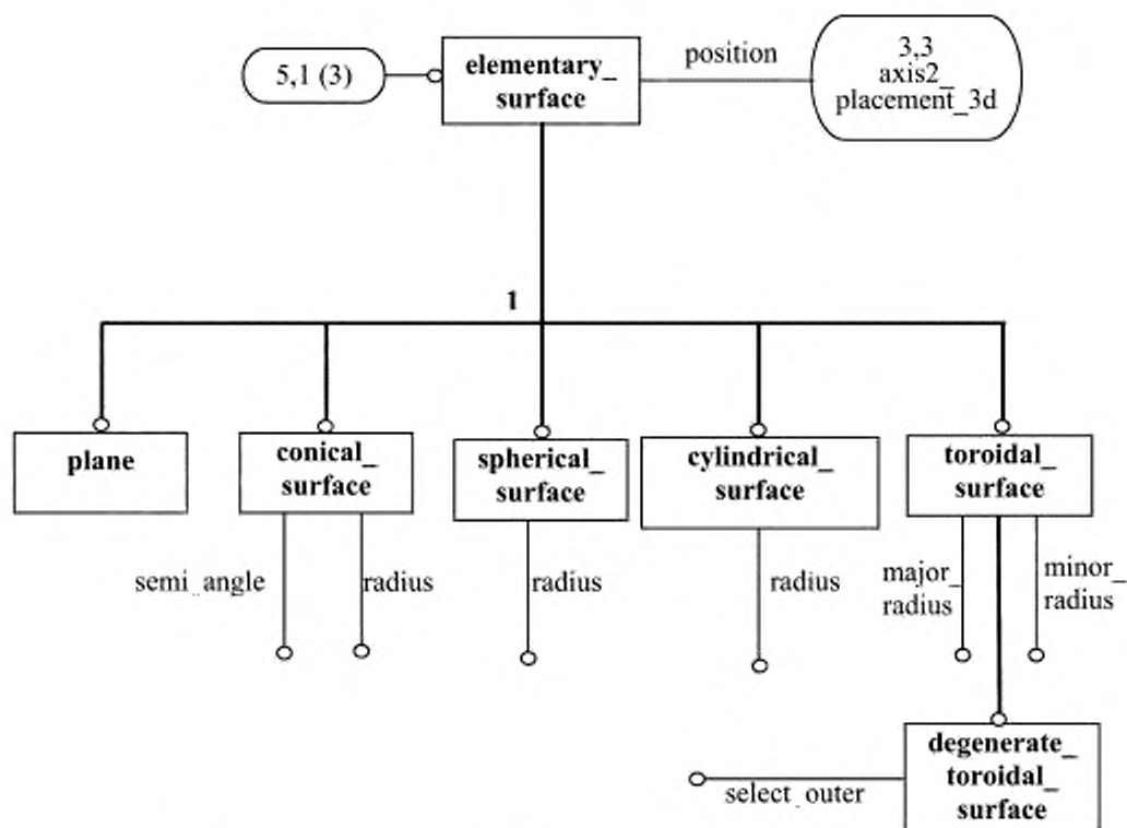
Рисунок D.5 — alc_topologically_bounded_surface — EXPRESS-G диаграмма 5 из 8
