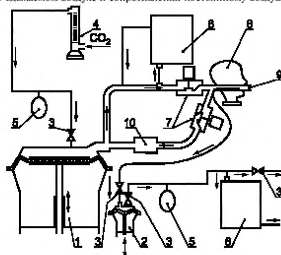
1 — дыхательная машина; 2 — вспомогательное «легкое»; 3 — односторонний клапан; 4 — измеритель потока; 5 — компенсатор; 6 — анализатор диоксида углерода; 7 — соленойдный клапан; 8 — голова-манекен; 9 — трубка отбора проб для вдыхаемого воздуха (см. рисунок 6); 10 — поглотитель диоксида углерода
