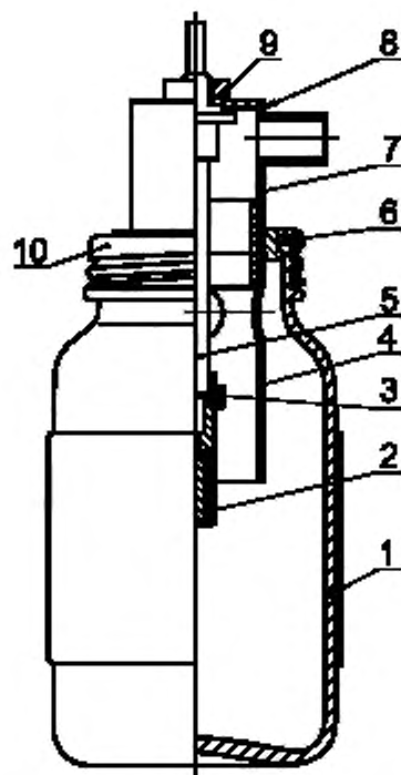
1 — стеклянный сосуд с навинчивающейся крышкой; 2 — соплло; 3 — волоконистая прокладка (наружный диаметр — 4,5 мм, внутренний диаметр — 2 мм, толщина прокладки — 0,8 мм); 4 — втулка; 5 — стержень; 6 — резиновая прокладка; 7 — головка втулки; 8 — резиновая прокладка (наружный диаметр — 25 мм, внутренний диаметр — 10 мм, толщина — 1,5 мм, уплотнитель для герметизации); 9 — гайка; 10 — навинчивающаяся крышка
