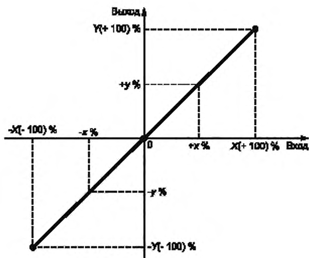
Рисунок 2 — Кривые передаточной функции
