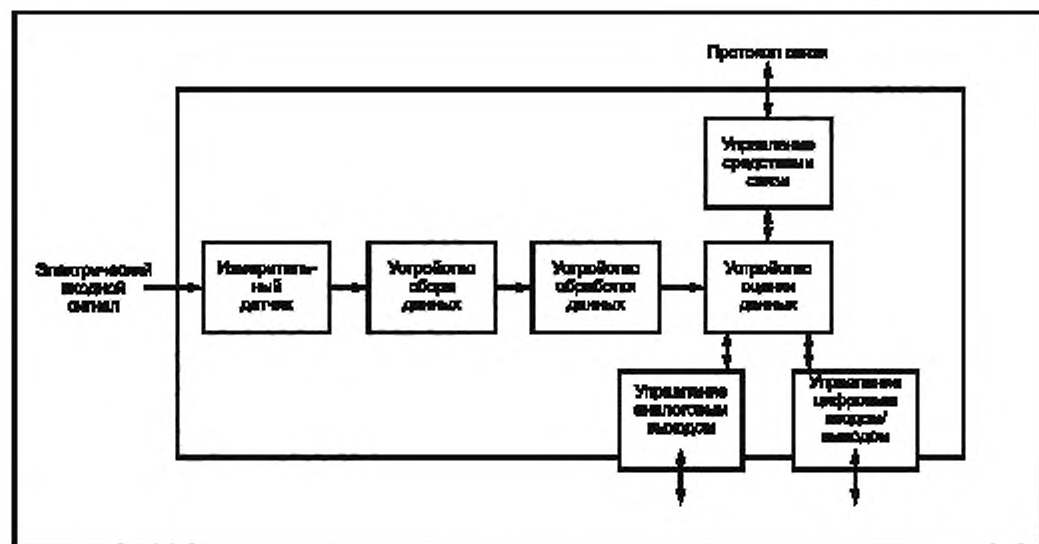
Рисунок 1 — Структура преобразователя
