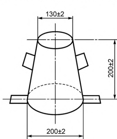
а) Форма-конус
