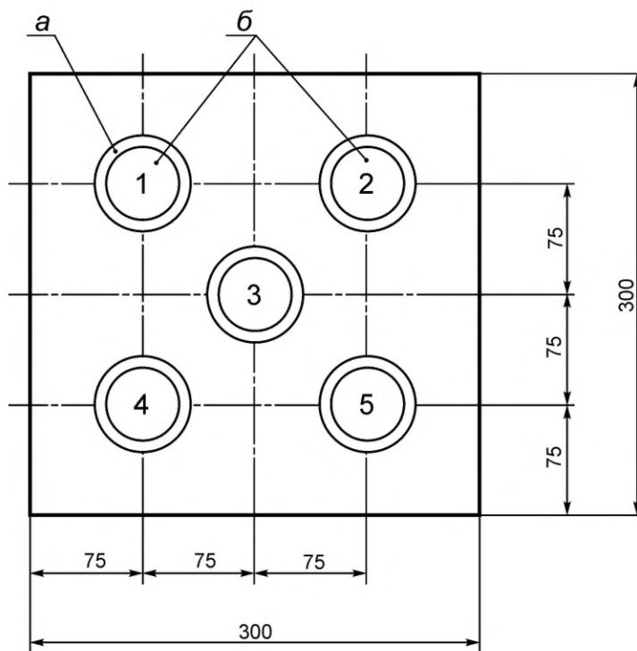
а — цилиндрический пропил; б — образец-керна; 1—5 — маркировка образцов-кернов
