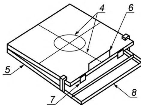
б) Трамбовка
