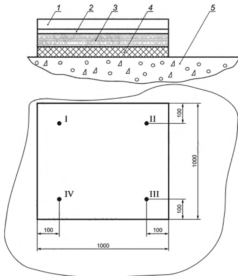
Рисунок 2 — Схема размещения точек на экспериментальном участке пола с покрытием по монолитной или сборной стяжке на теплозвукоизолирующем слое
