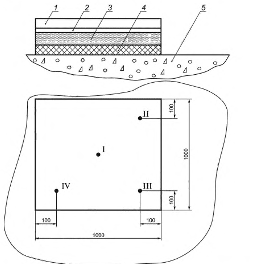
1 — покрытие пола; 2 — клеевая прослойка (при наличии в конструкции пола); 3 — монолитная или сборная стяжка; 4 — клеевая прослойка (при наличии в конструкции пола); 5 — бетонный подстилающий слой или плита перекрытия; ● I — ● IV — точки установки деформатора
