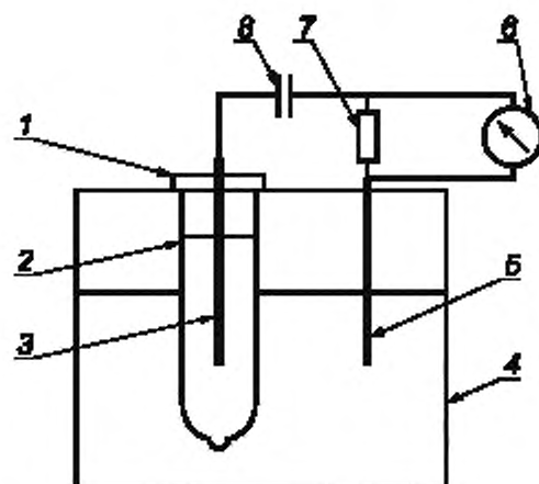
1 — опора (см. рисунок Ж.3); 2 — презерватив, наполненный электролитом и закрепленный на опоре; 3 — электрод, прикрепленный к опоре; 4 — контейнер с электролитом; 5 — электрод; 6 — вольтметр; 7 — резистор сопротивлением 10 кОм; 8 — источник стабилизированного постоянного тока напряжением 10 В
