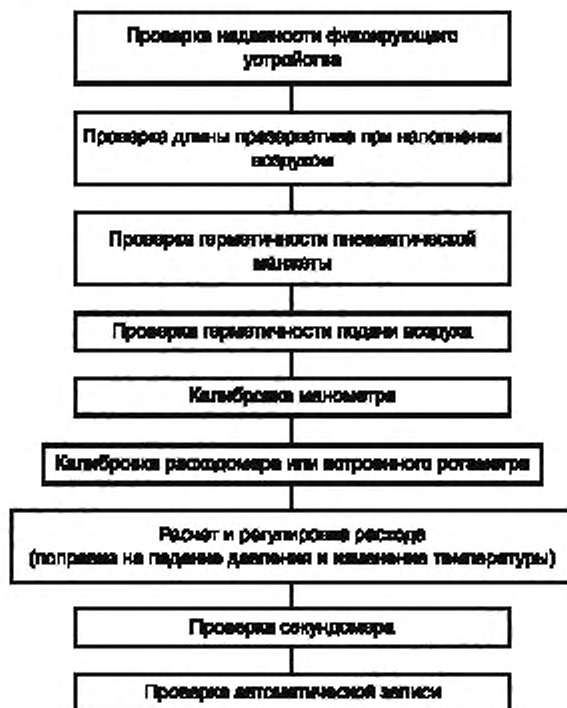
Рисунок I.1 — Последовательность проведения калибровки
