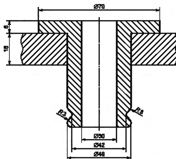
Рисунок Ж.3 — Пример приспособления для крепления презерватива на опоре
