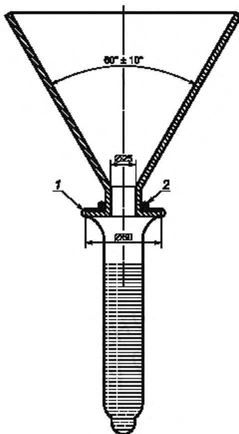
1 — закругленная кромка; 2 — резиновое кольцо
