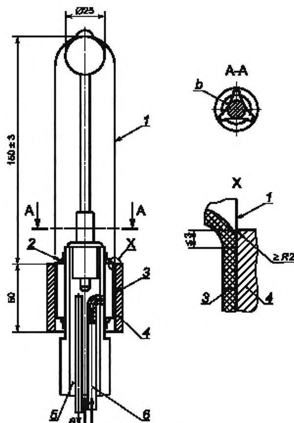
1 — презерватив; 2 — корд; 3 — гибкая пневматическая манжета; 4 — фиксирующее кольцо; 5 — впуск воздуха для испытания; 6 — впуск воздуха для фиксации презерватива; а — к устройству измерения давления; б — области, открытые для потока воздуха
