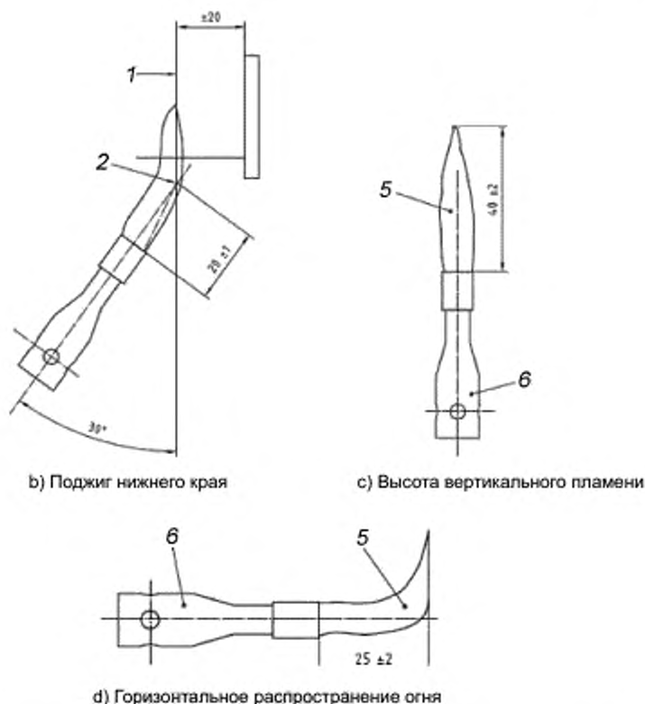
1 — образец ткани; 2 — номинальная точка распространения пламени; 3 — палец крепления; 4 — крепежная стойка; 5 — пламя; 6 — горелка
