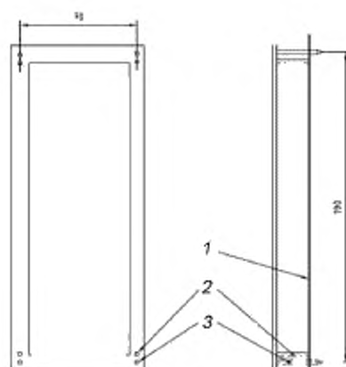
1 — образец для испытаний; 2 — разделительная ножка; 3 — палец крепления
