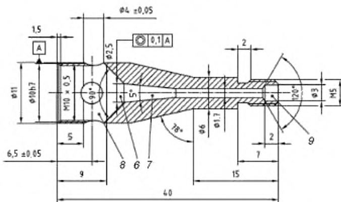
d) Трубка горелки
