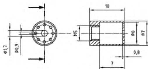
с) Стабилизатор пламени
