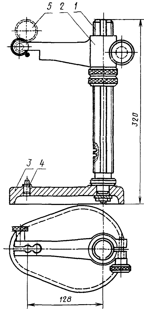
1—стойка; 2—кронштейн; 3—нижняя опора; 4—конусообразный выступ; 5—индикатор
