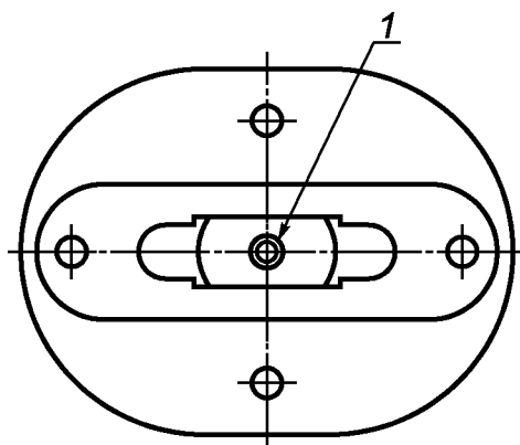
1 — пробоотборный порт
