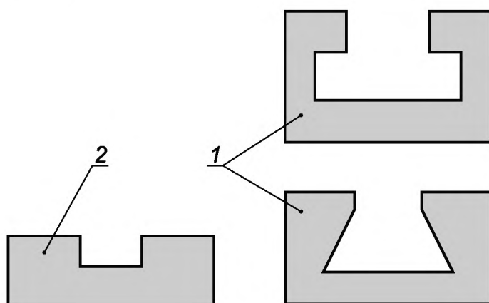
Рисунок 21 — Примеры формы паза приспособления для установки поперечной направляющей линейки на круглопильных универсальных станках
