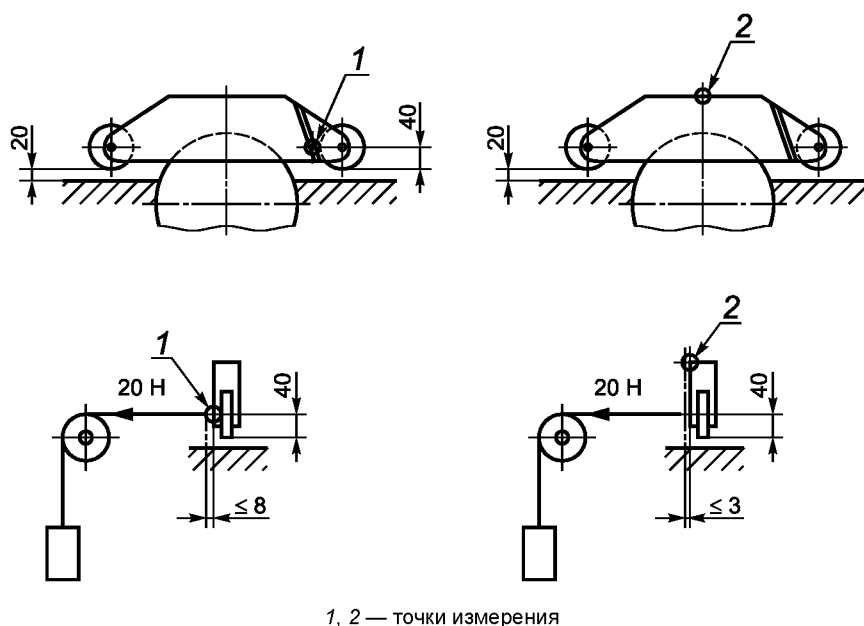
Рисунок F.2 — Испытание на устойчивость ограждений дисковой пилы на подающих роликах, установленных отдельно от расклинивающего ножа
