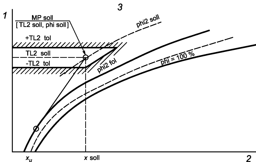
1 — массовая энтальпия воздуха h ; 2 — абсолютная влажность окружающего воздуха x\phi ; 3 — диаграмма Молльера
