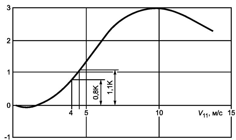
Рисунок А.2 — Пример воздействия ветра на градирню с противотоком и естественной тягой
