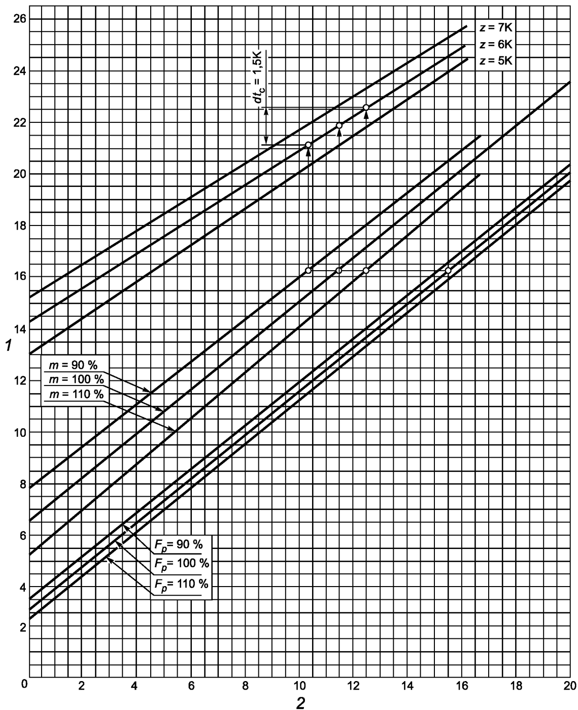
Рисунок А.4 — Испарительная вентиляторная градирня
