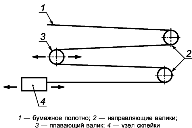
Рисунок 4 — Устройство автосклейки
