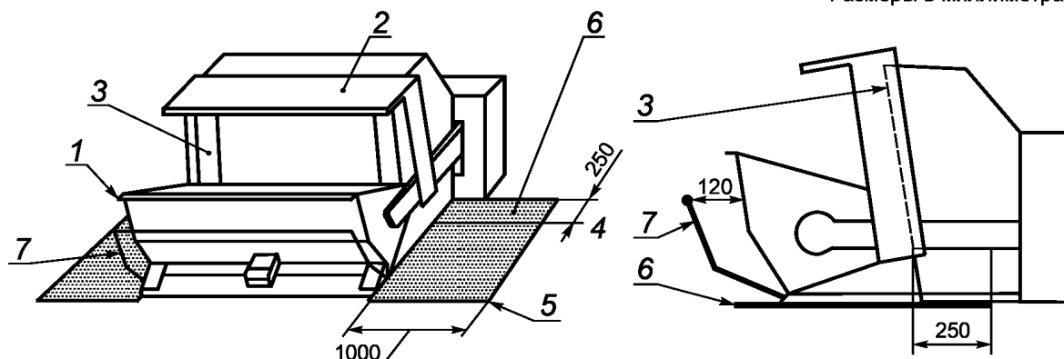
1 — отключающая планка; 2 — ограждение автоматического отключения; 3 — плоскость высечки; 4 — нижний край плоскости высечки; 5 — передний край подвижного тигля; 6 — коврик, реагирующий на надавливание; 7 — коленчатый рычаг (скоба)
