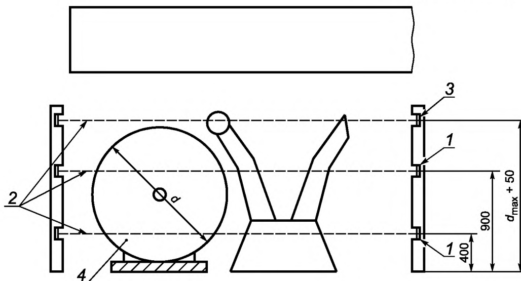
1 — ЭЧПУ; 2 — фотоэлектрический луч ЭЧПУ; 3 — дополнительное ЭЧПУ; 4 — рулон материала
