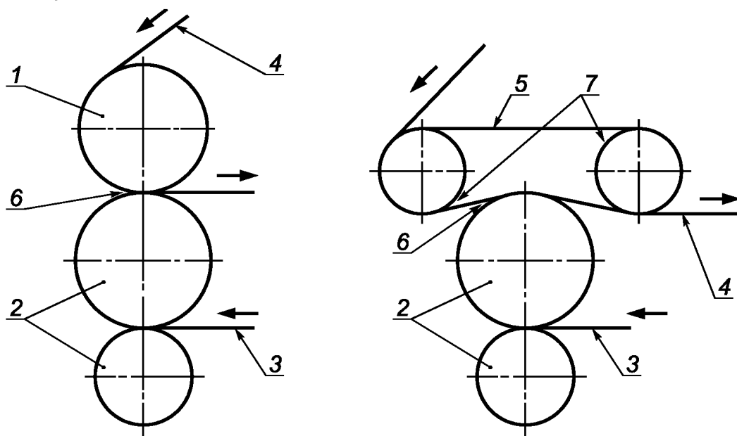
Прижимной вал
