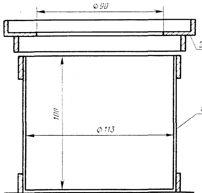
Прибор для определения объемной массы растворной смеси
