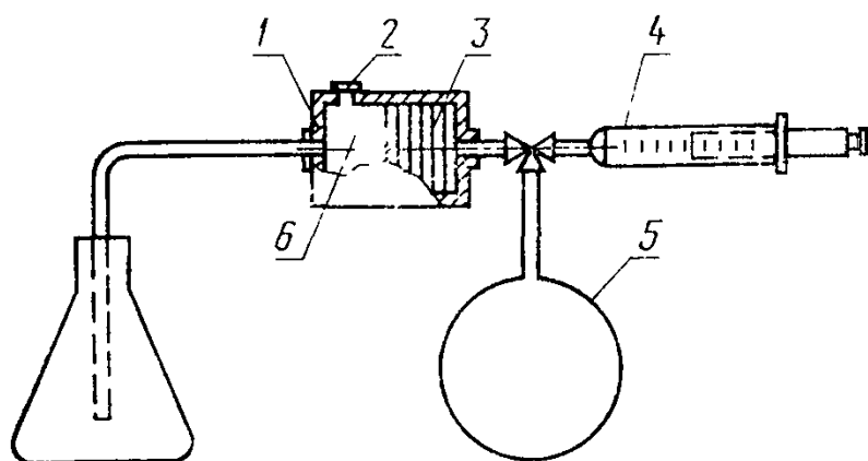
1—пламепреградитель; 2—предохранительная мембрана, 3—пластинки из спеченного стекла (перегородки); 4—термостатический шприц, 5—резервуар с газом, 6—предкамера
