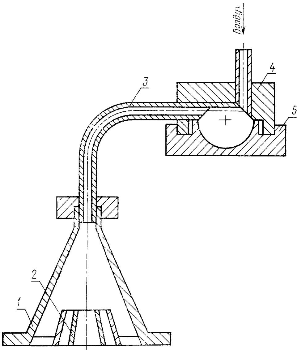
1—корпус; 2—рассекатели 3—патрубок, 4—корпус форкамеры, 5—доннышко Черт. 11
