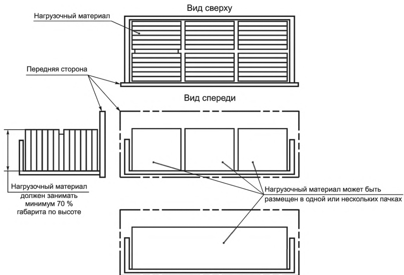
Рисунок 9 — Конфигурация нагрузки для ящиков (ширина больше глубины) с дном, воспринимающим нагрузку
