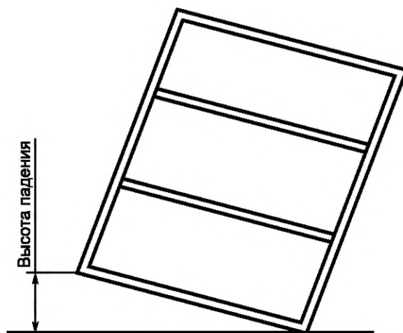
Рисунок 4 — Испытание картотек на прочность
