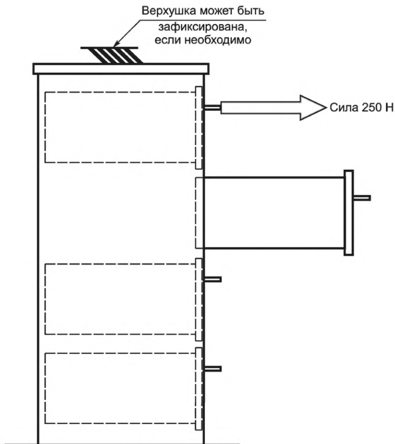
Рисунок 6 — Испытание на прочность блокирующего устройства
