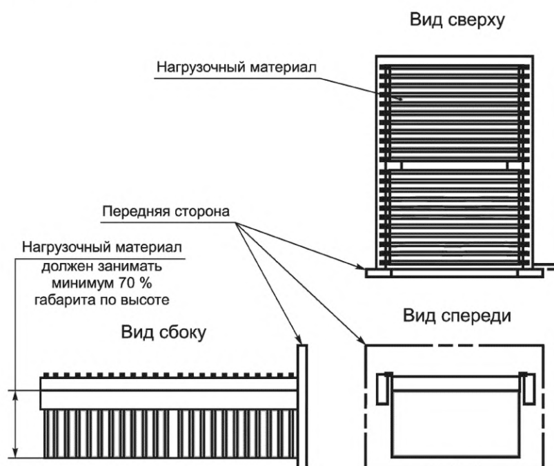
Рисунок 10 — Конфигурация нагрузки для ящиков (глубина больше ширины) без дна
