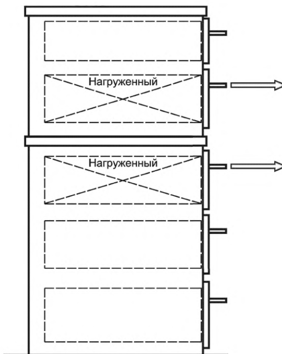
Рисунок 3 — Испытание на устойчивость картотек при установке друг на друга
