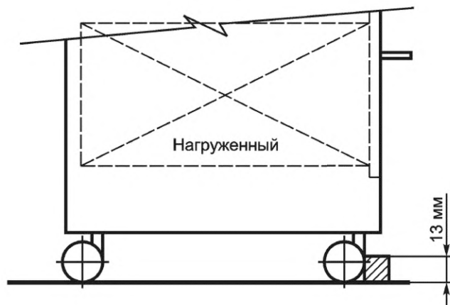
Рисунок 1 — Установка картотек для проведения испытаний
