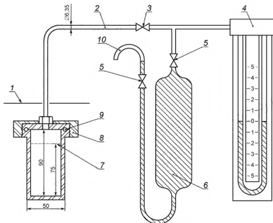
1 – уровень масляной ванны; 2 – трубопровод из нержавеющей стали; 3 – вентиль; 4 – ртутный манометр 25 см; 5 – вентили; 6 – газосборник объемом 250 см 3 , заполненный водой; 7 – уровень пробы смазки; 8 – автоклав; 9 – силиконовое уплотнительное кольцо; 10 – трубка для измерения вытесненного объема
