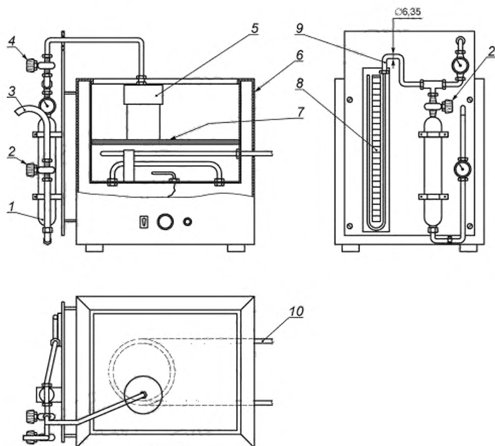
1 — газосборник объемом 250 см 3 , заполненный водой, 2 — вентиль; 3 — трубка для измерения вытесненного объема; 4 — вентиль; 5 — автоклав; 6 — ванна с постоянной температурой; 7 — полка; 8 — ртутный манометр 25 см; 9 — трубопровод из нержавеющей стали, 10 — подвод воды 66 °С (см. сноску а к рисунку Н.2)
