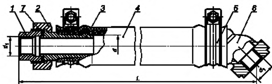
1 — гайка соединительная; 2 — гайка накидная; 3 — наконечник; 4 — рукав по ГОСТ 1335; 5 — хомут; 6 — наконечник; 7 — прокладка
