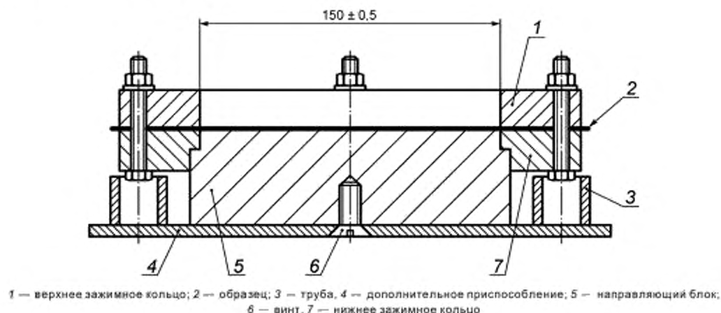
а) Пример зажимных колец, использование направляющего блока
