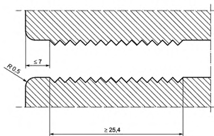
б) Пример деталей зубчатых поверхностей
