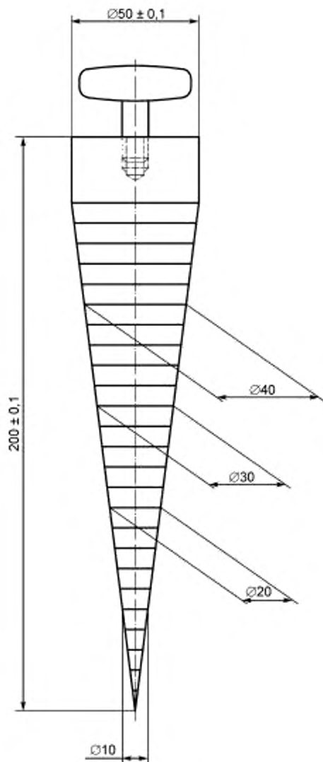
Рисунок 4 — Пример измерительного конуса
