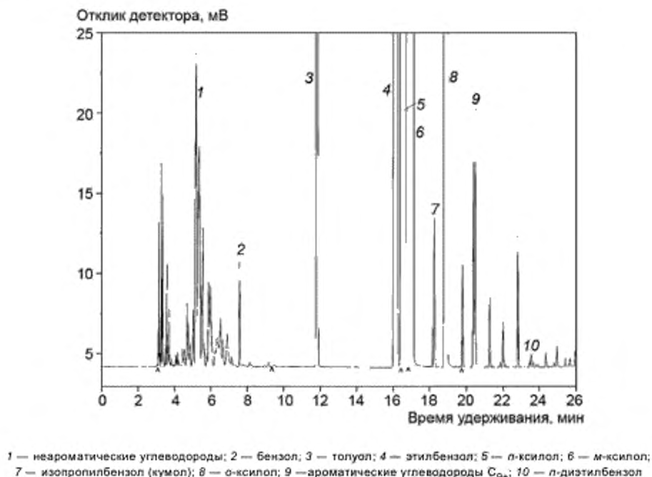
Рисунок 3 — Типичная хроматограмма смеси ксилолов по ASTM Д 5211
