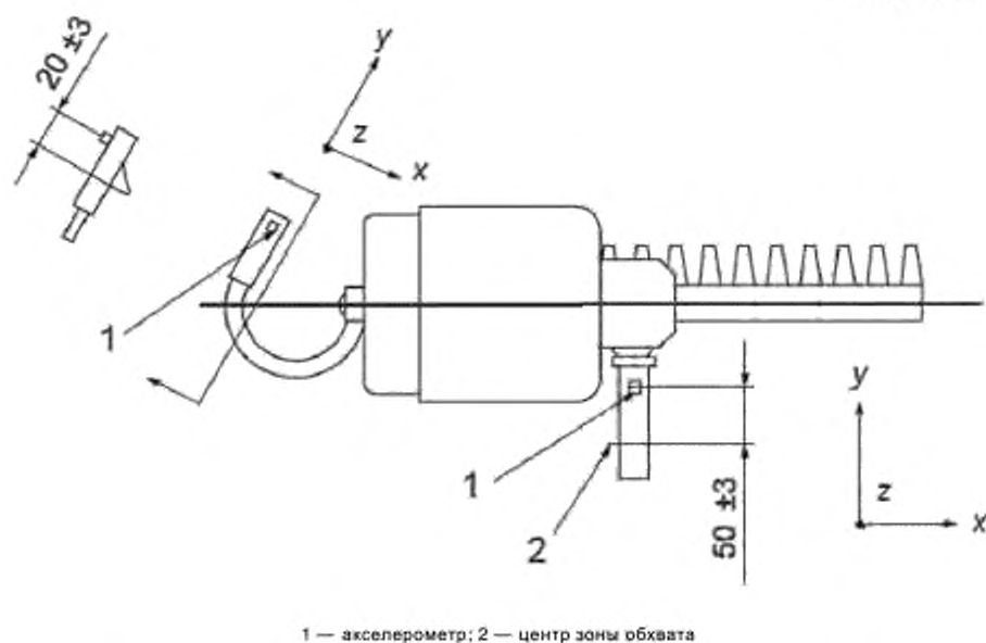
Рисунок D.2 — Направления измерений и точки крепления акселерометров на машинах с поперечными рукоятками
