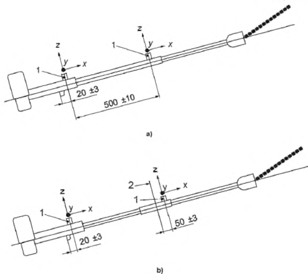
Рисунок D.3 — Направления измерений и точки крепления акселерометров на машинах дальней досягаемости
