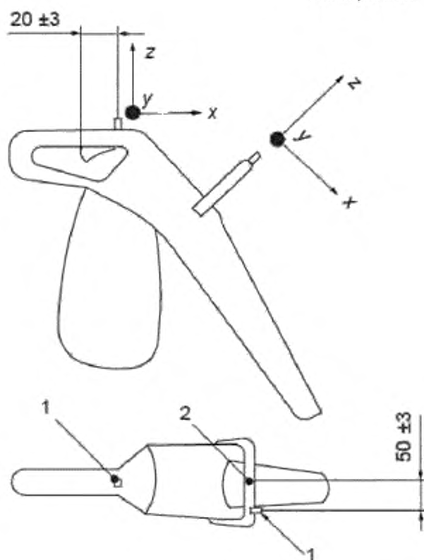
Рисунок Е.3 — Направления измерений и точки крепления акселерометров на двухручном пылесосе/воздуходувке
