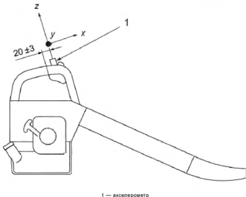
1 — акселерометр
