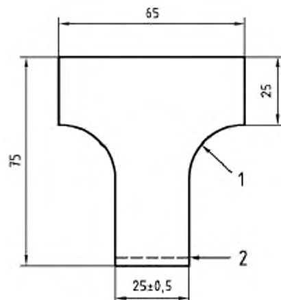
Рисунок 2 — Образец для испытания
