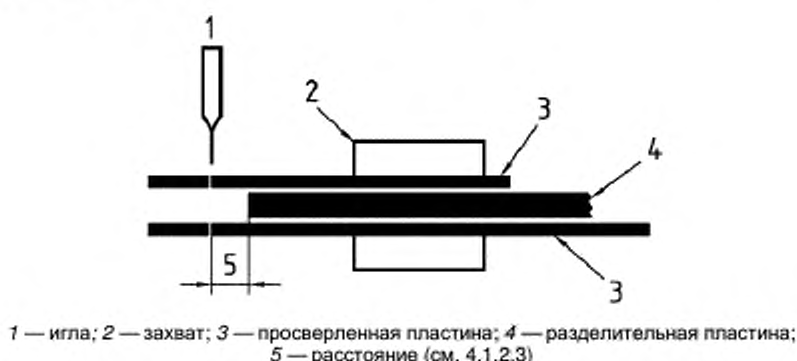
Рисунок 1 — Схематическое изображение устройства с иглой
