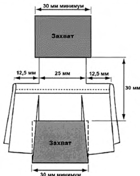
Рисунок 4 — Испытуемый образец в захватах
