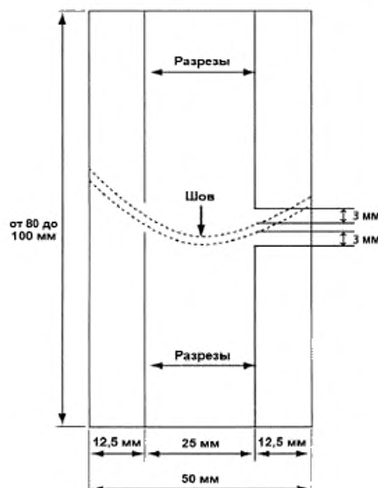
Рисунок 3 — Образец, вырезанный из готового изделия
