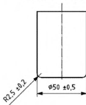
Рисунок 1 — Схема штампа
