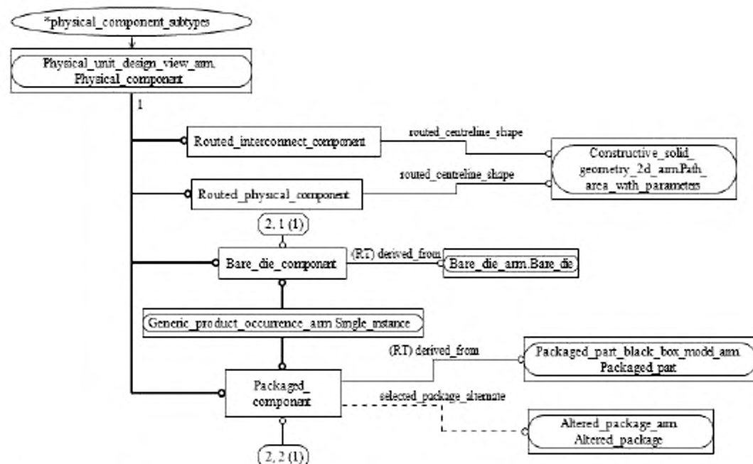
Рисунок С.3 — Представление ПЭМ на уровне объектов в формате EXPRESS-G. Диаграмма 2 из 3
