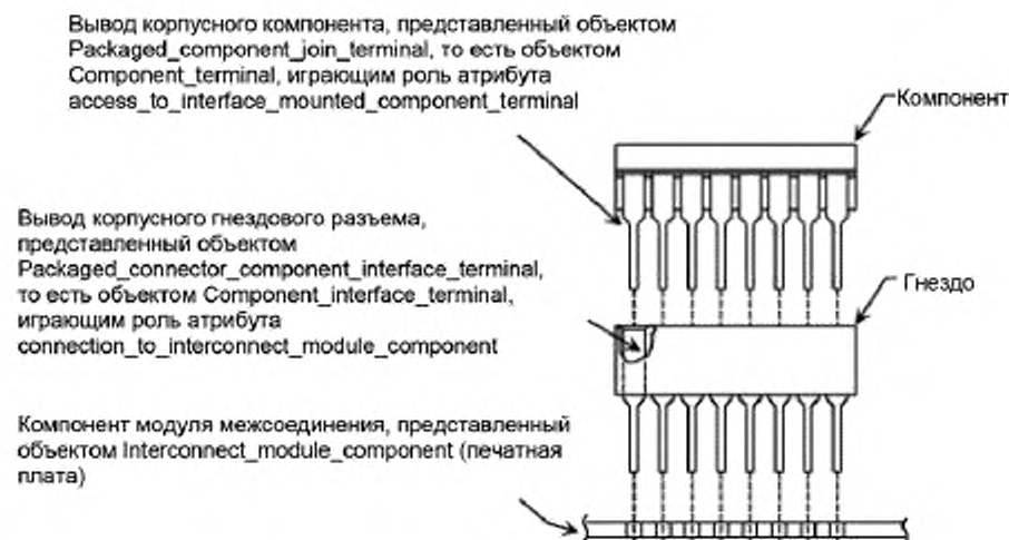
Рисунок 3 — Вывод корпусного компонента, представленный объектом Packaged_component_join_terminal
