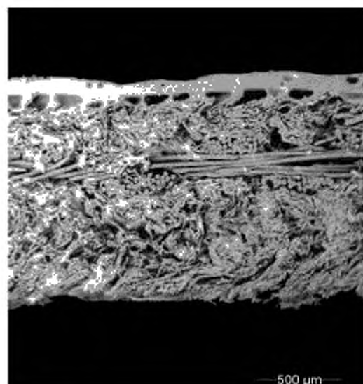
Рисунок А.11 — Сечение текстильного материала, покрытого коженными волокнами
