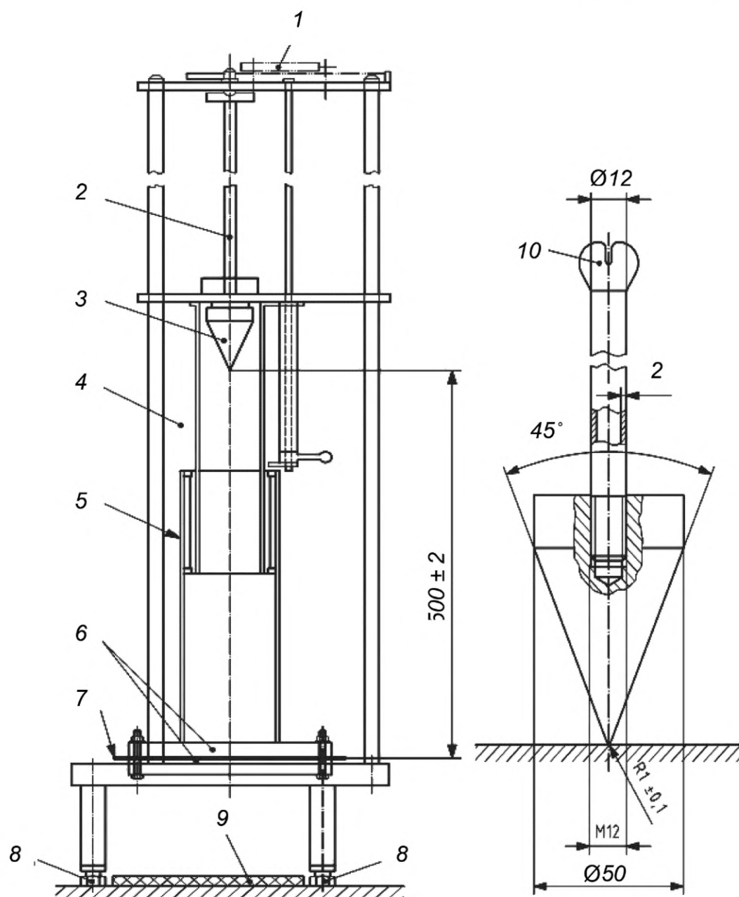
1 — головная часть спускового механизма соответствующего лабораторного оборудования; 2 — направляющий шток; 3 — испытательный конус; 4 — металлический экран; 5 — защитный экран; 6 — зажимная система (обойма); 7 — образец геосинтетического материала; 8 — регулировочный винт; 9 — амортизирующий слой; 10 — верхняя часть испытательного конуса
