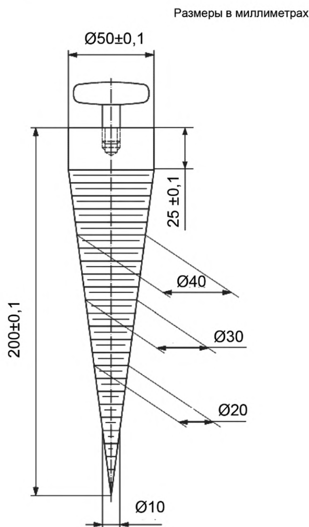
Рисунок 3 — Измерительный конус
