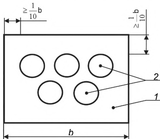
Рисунок 4 — Схема отбора испытываемых образцов
