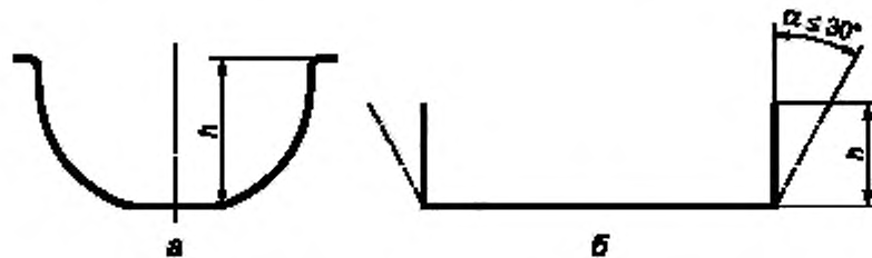
Рисунок 9 — Профили горки
