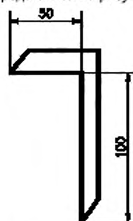
Рисунок А.3 — Шаблон для измерения профиля горки
