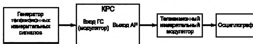
Рисунок 7.2 — Структурная схема измерения импульсной характеристики канала распределения (К-фактора)
