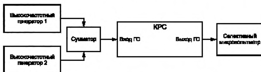
Рисунок 7.1 — Структурная схема для определения неравномерности АЧХ в канале распределения радиосигнала вещательного телевидения
