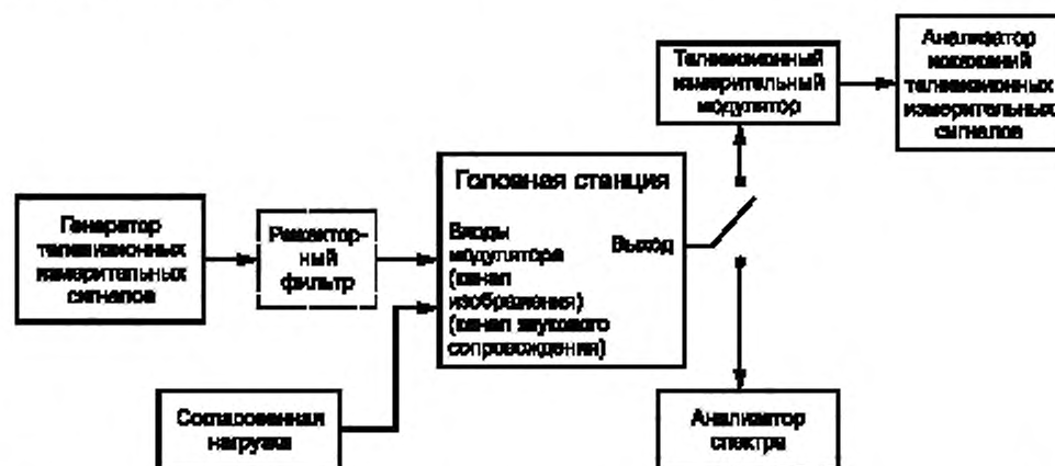
Рисунок 7.18 — Структурная схема для определения отношения радиосигнала к одночастотной помехе комбинационных частот третьего порядка IMA_{(3/K)}
