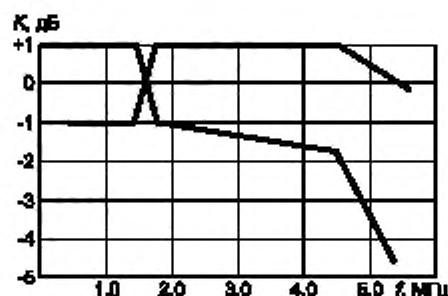
Рисунок В.1 — Поле допуска сквозной АЧХ канала изображения
