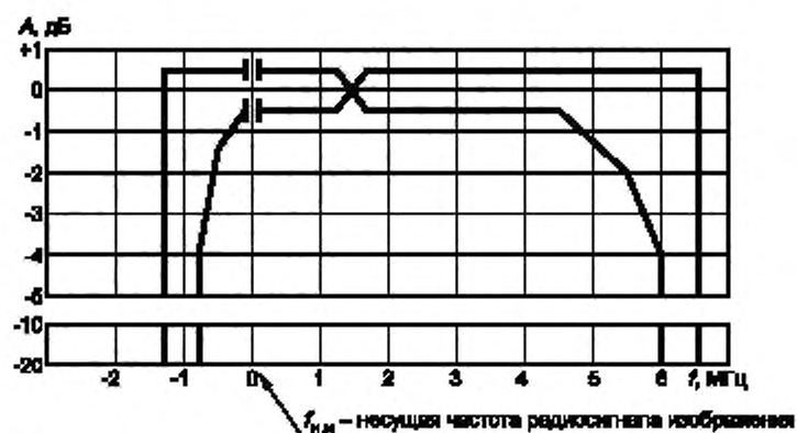
Рисунок Б.1 — Поле допуска характеристики боковых полос в полосе частот от f_{н.и} - 1,25 МГц до f_{н.и} + 6,5 МГц
