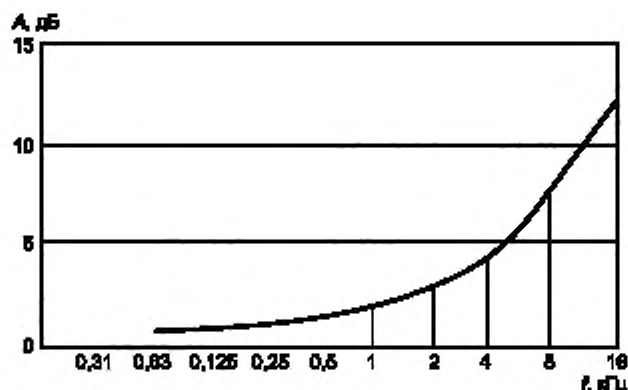
Рисунок 5.2 — АЧХ цепи предусылажения с постоянной времени 50 мс
