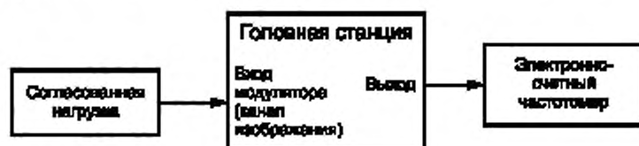
Рисунок 7.22 — Структурная схема для определения отклонения несущей частоты радиосигнала изображения от номинального значения
