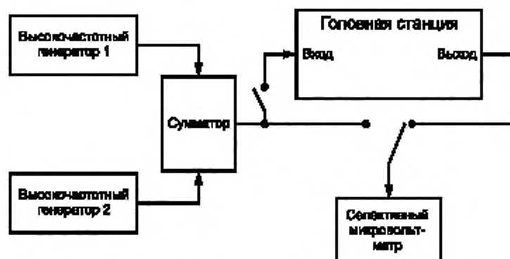
Рисунок 7.13 — Структурная схема для определения отношения радиосигнала изображения к побочным помехам, неравномерности АЧХ в канале распределения и избирательности канального усилителя (конвертора) ГС
