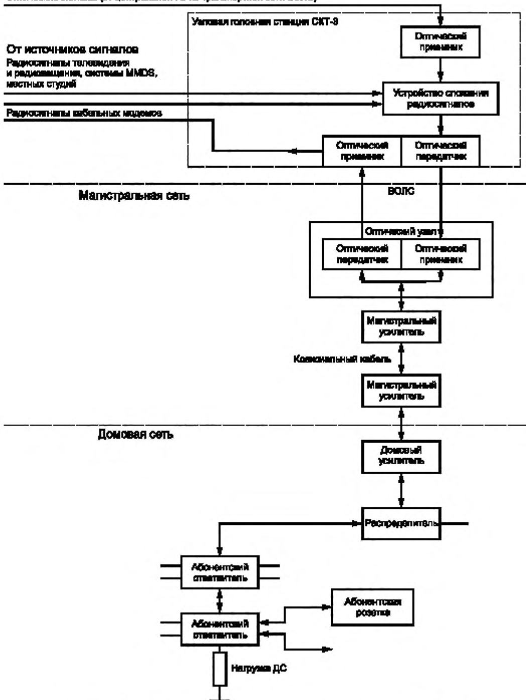
Рисунок 4.3 — Структурная схема городской кабельной распределительной сети SKT-3
