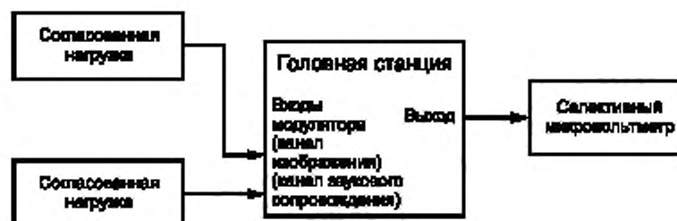
Рисунок 7.19 — Структурная схема для определения отношения радиосигнала изображения к побочным помехам, разности уровней напряжения радиосигналов изображения и звукового сопровождения, отношения радиосигнала изображения к шуму в полосе частот канала изображения
