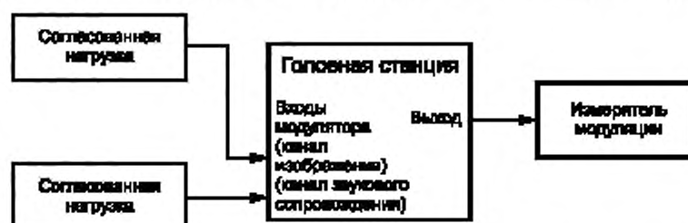
Рисунок 7.24 — Структурная схема для определения отношения сигнала к фоновой помехе
