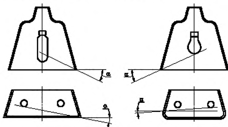
Рисунок А.5 — Защитные углы для различных типов светильников, лампы которых полностью или частично видны (или их отражение), когда на них смотрят под критическим углом
