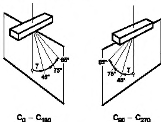
Рисунок А.4 — Плоскости C и углы \gamma , для которых должно быть проверено распределение яркости
