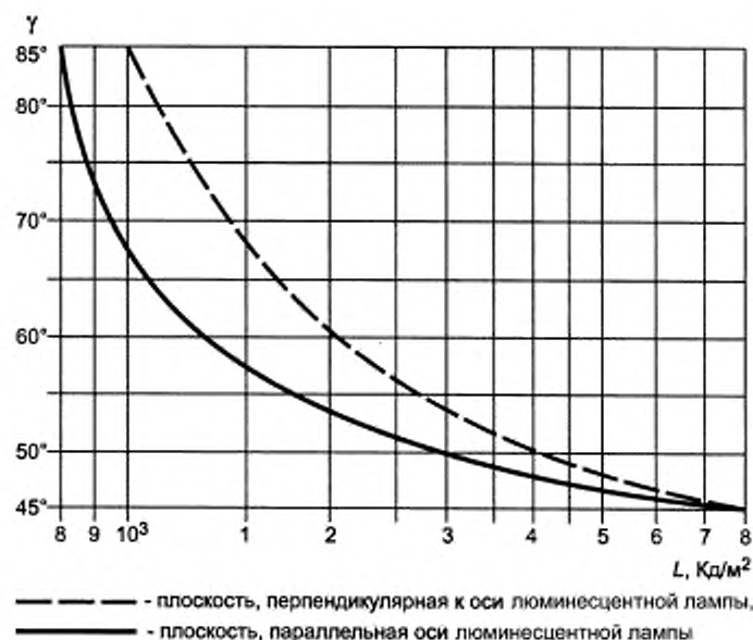
Рисунок А.6 — Кривые яркости для примеров 1 и 2
