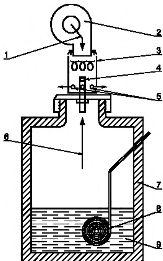
1 — поступающий воздух; 2 — центробежный вентилятор; 3 — дисперсионная камера; 4 — форсунка; 5 — пар с воздухом; 6 — пар; 7 — изолированный контейнер; 8 — нагревательный элемент; 9 — вода
