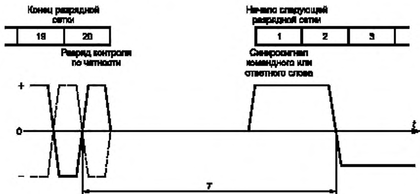
Рисунок 10 — Измерение временных пауз T в сообщениях
