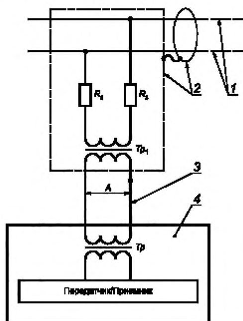
Tr — трансформатор гальванической развязки; Tr_1 — согласующий трансформатор; R_1 — защитные резисторы; 1 — магистральная шина; 2 — экран; 3 — шлейф; 4 — устройство интерфейса
