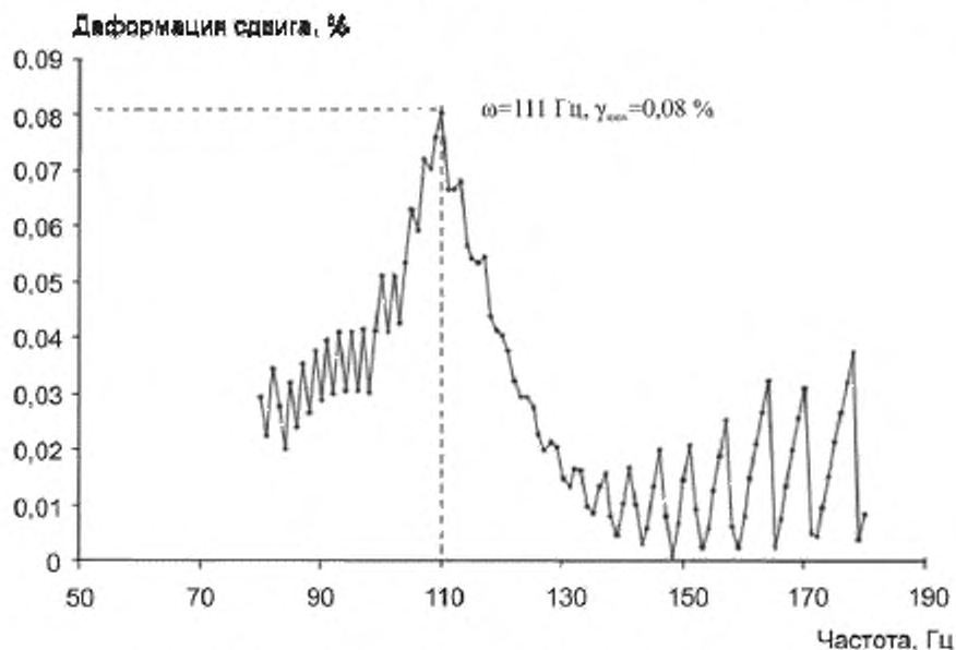
Рисунок Л.1 – Пример резонансной кривой образца грунта
