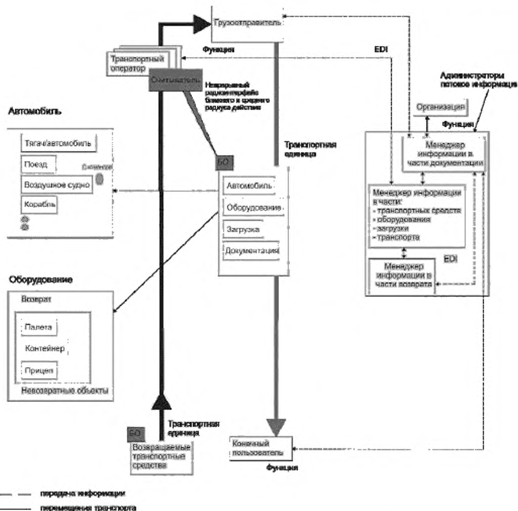
Рисунок 2 — Концептуальный вид системы AVI/AEI
